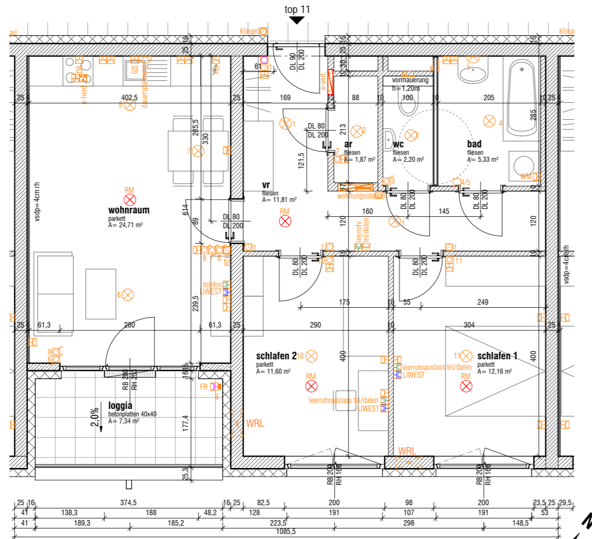
Grundriss M=1:75
