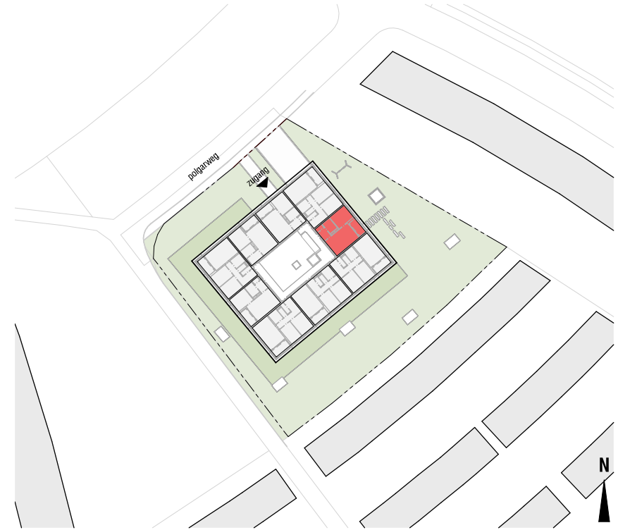
Lageplan M=1:750
