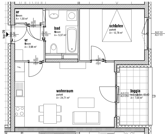
Grundriss M=1:75
