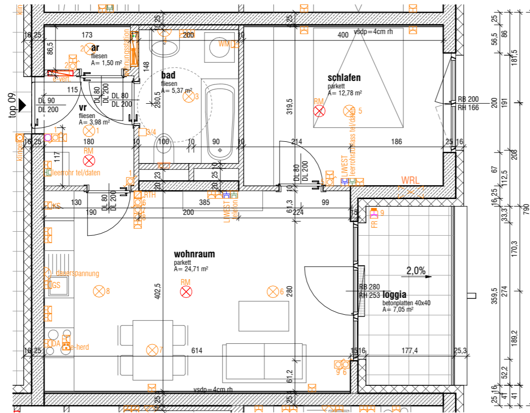
Grundriss M=1:75
