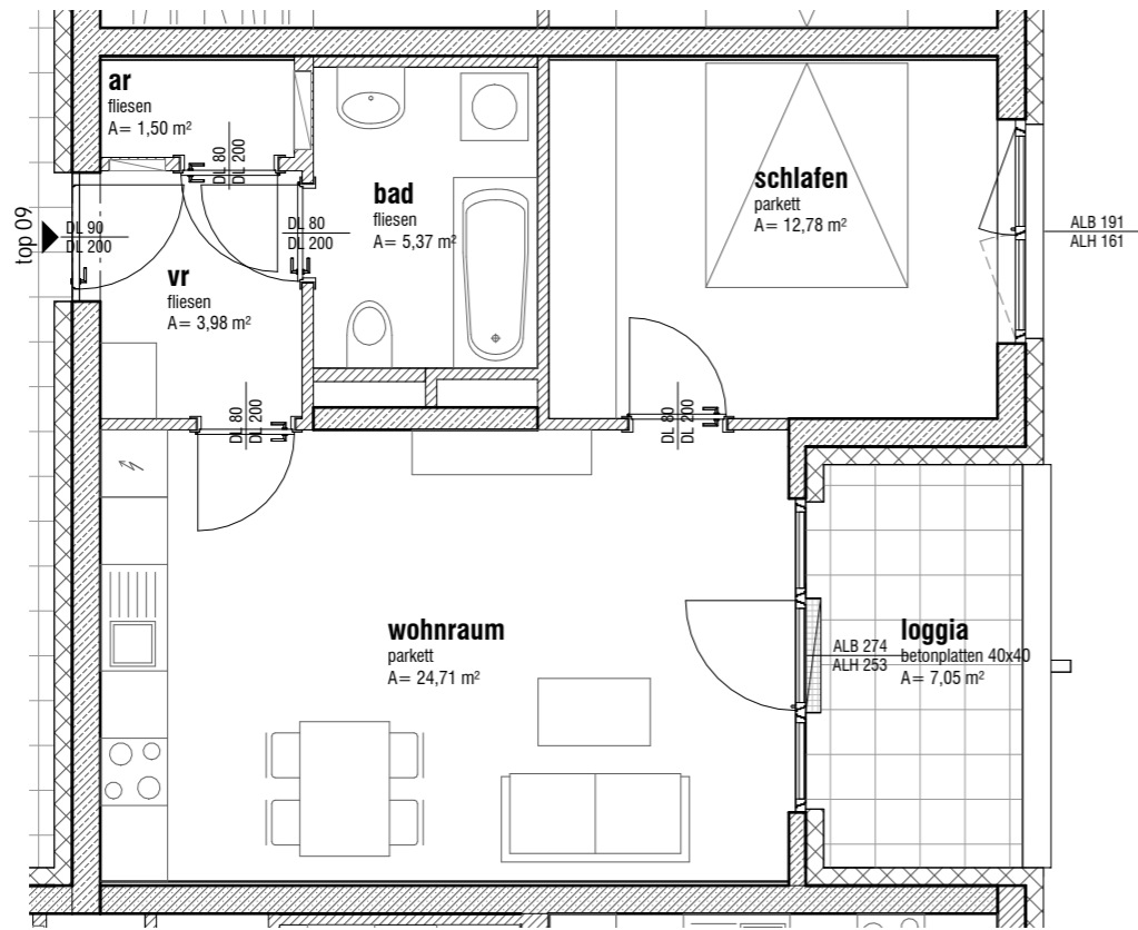
Grundriss M=1:75
