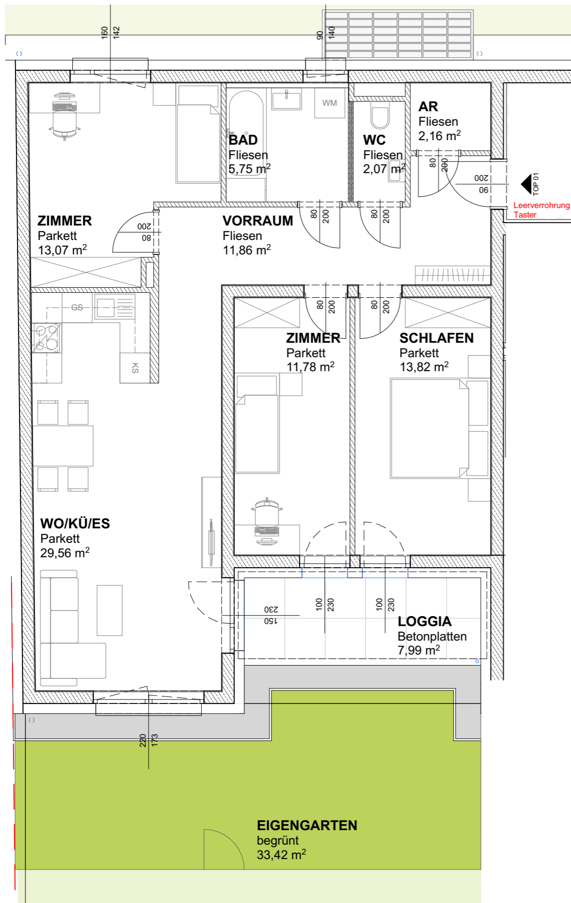
GRUNDRISS | M 1:75
