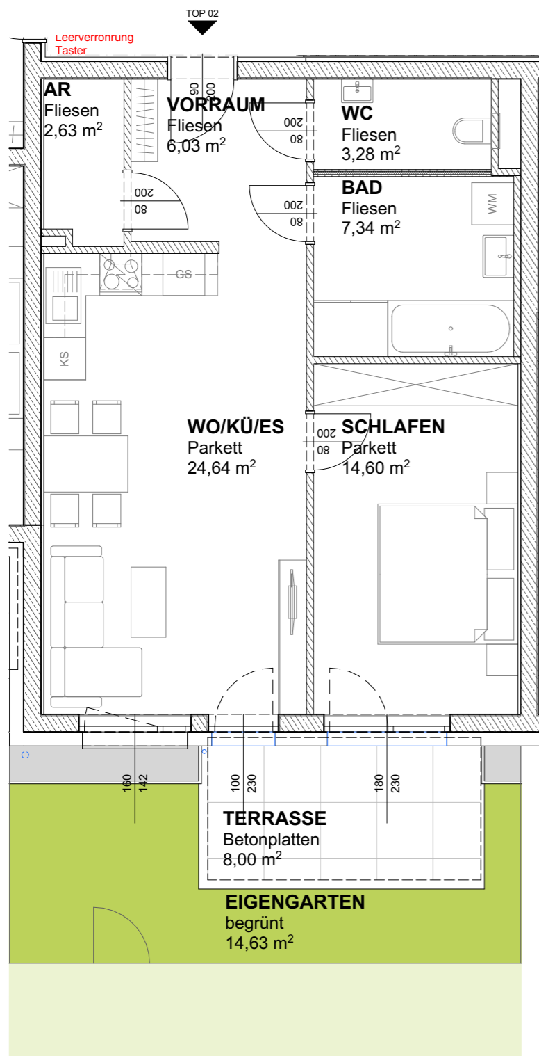
GRUNDRISS | M 1:75
