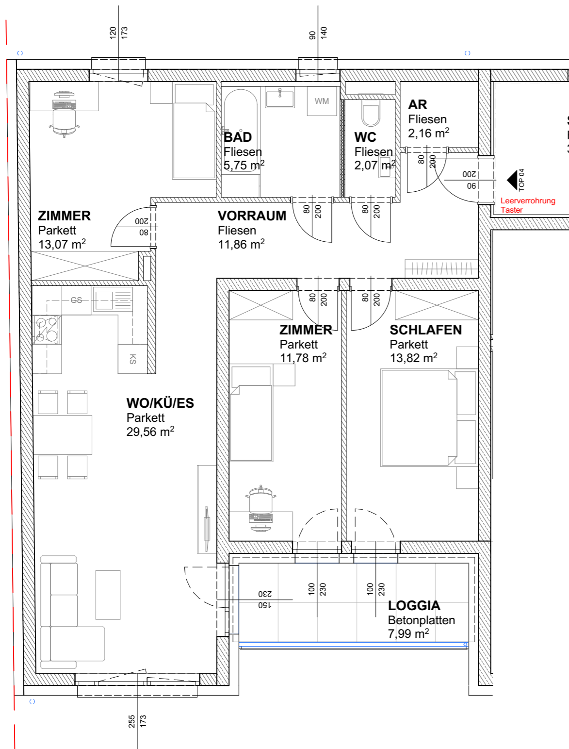
GRUNDRISS | M 1:75
