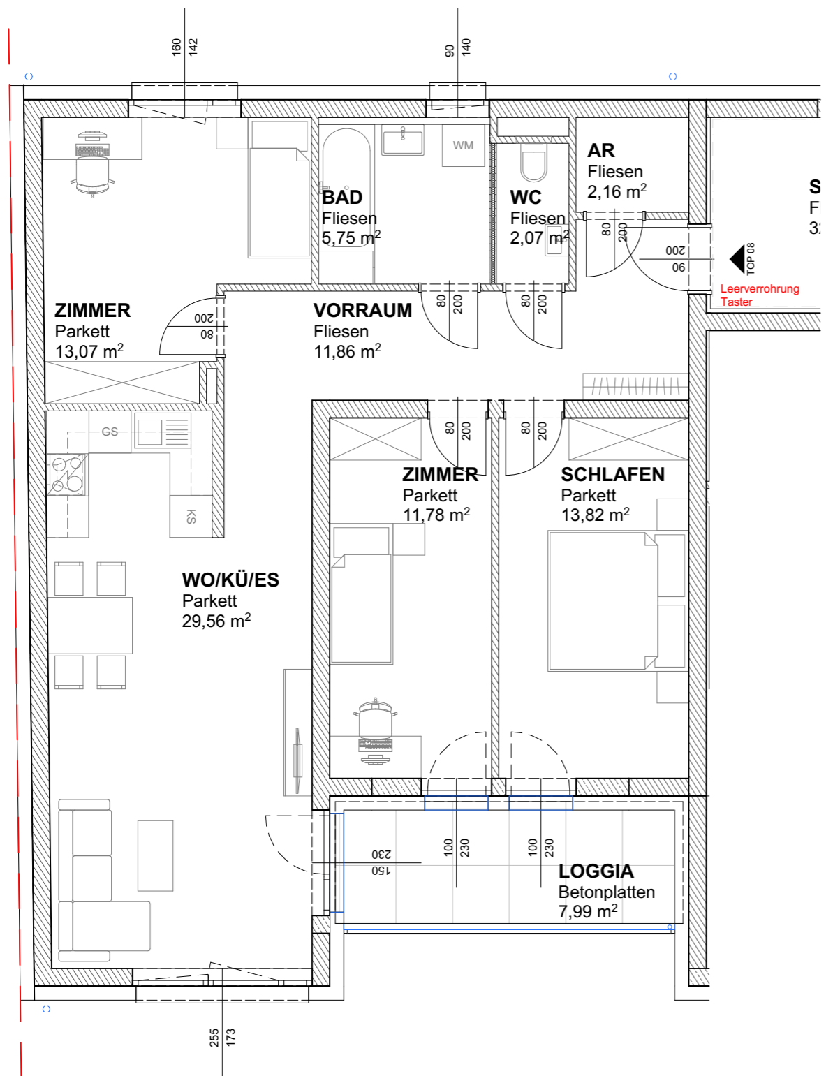
GRUNDRISS | M 1:75
