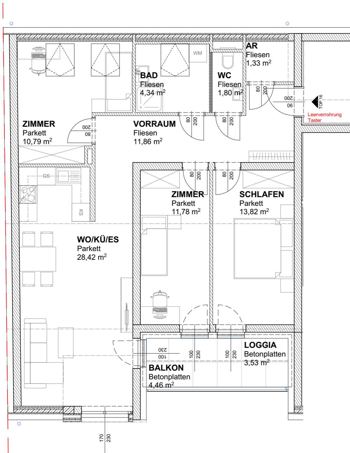
GRUNDRISS | M 1:75
