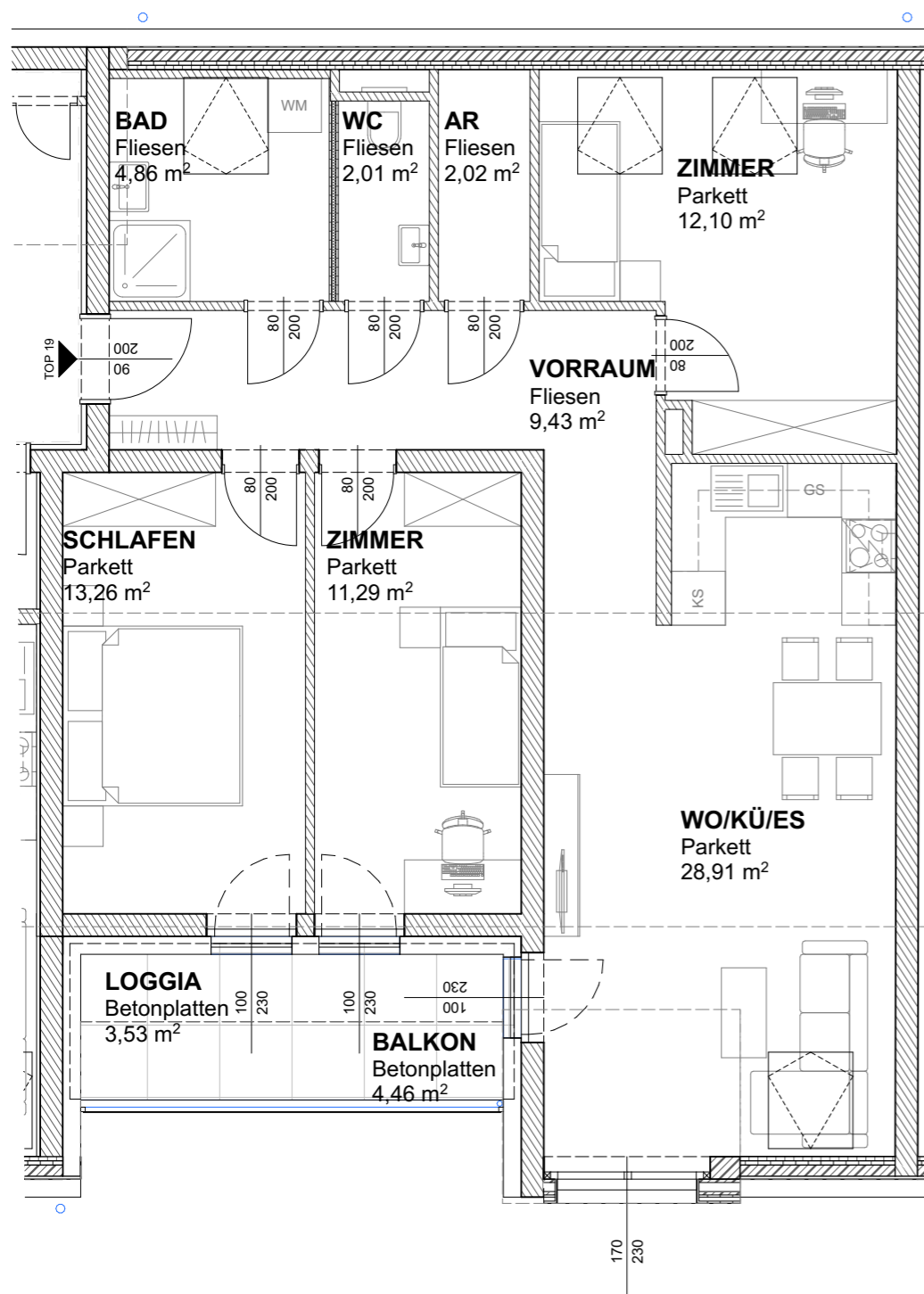
GRUNDRISS | M 1:75
